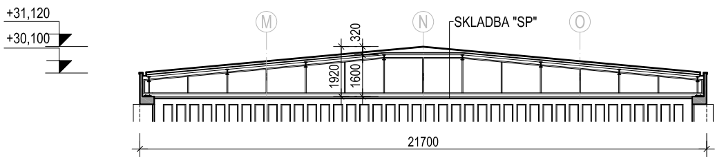
ŘEZ I - I' 1 : 200
