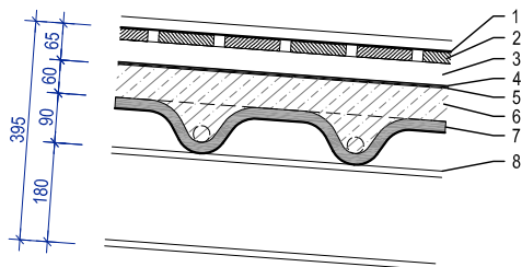
DETAIL STŘ. PLÁŠTĚ VE SKLADBĚ "SP" Popis jednotlivých vrstev skladeb viz. textová zpráva
