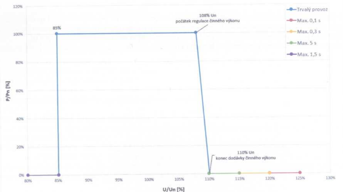
Snížení činného výkonu v závislosti na síťovém napětí
