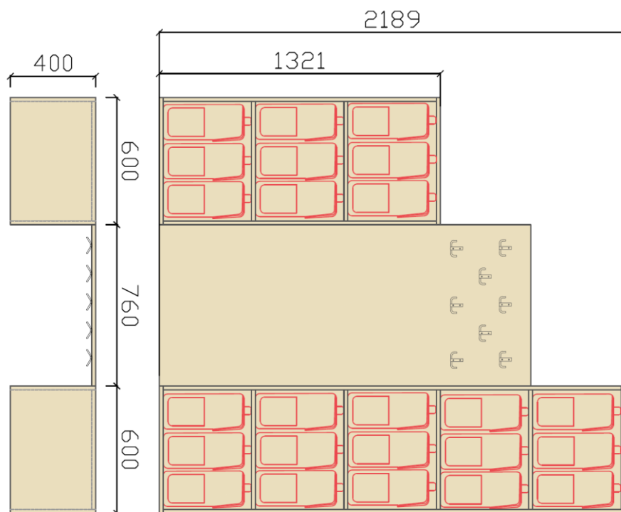
Nákres pro položku Úložný prostor na aktovky do učebny Učebna přírodních věd (v podkroví) a Učebna informatiky (v podkroví), míry uvedeny v mm
