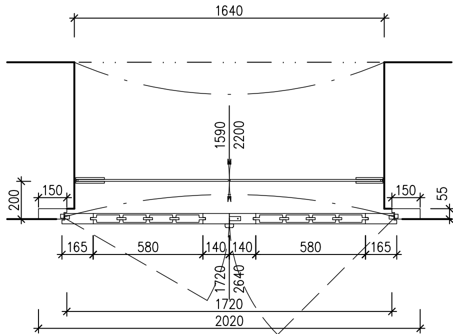
POHLED FASÁDNÍ
