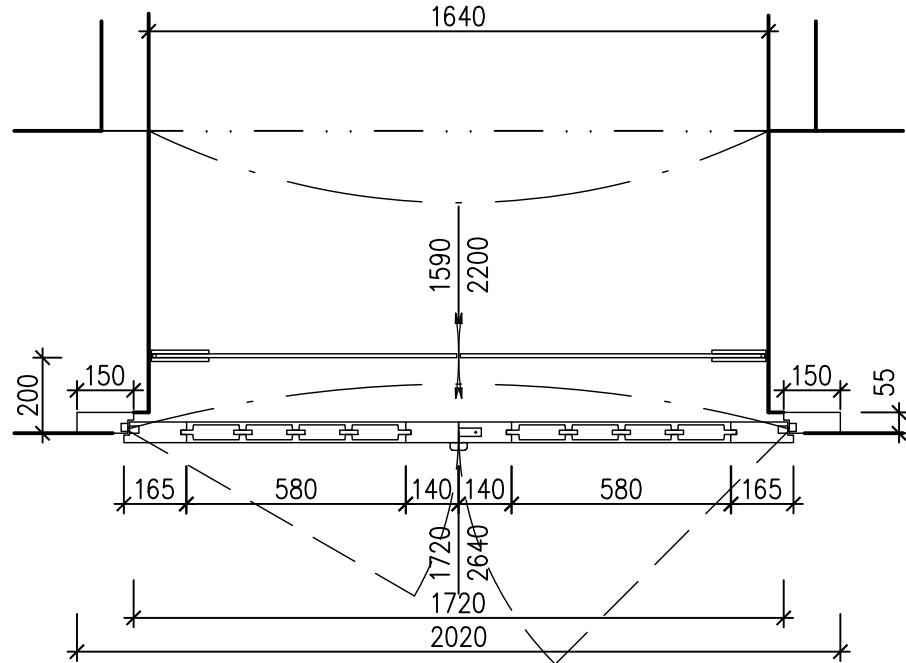
POHLED FASÁDNÍ
