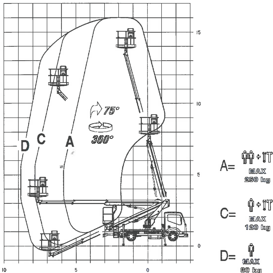
Obr. - pracovní diagram - boční dosah se automaticky nastaví dle zatížení klece.
